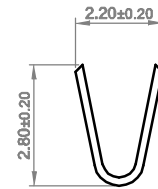
Sec:A-A
