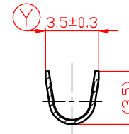
SEC.B-B
