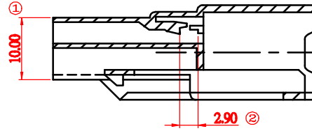
SEC A-A
