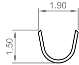
Sec:B-B
